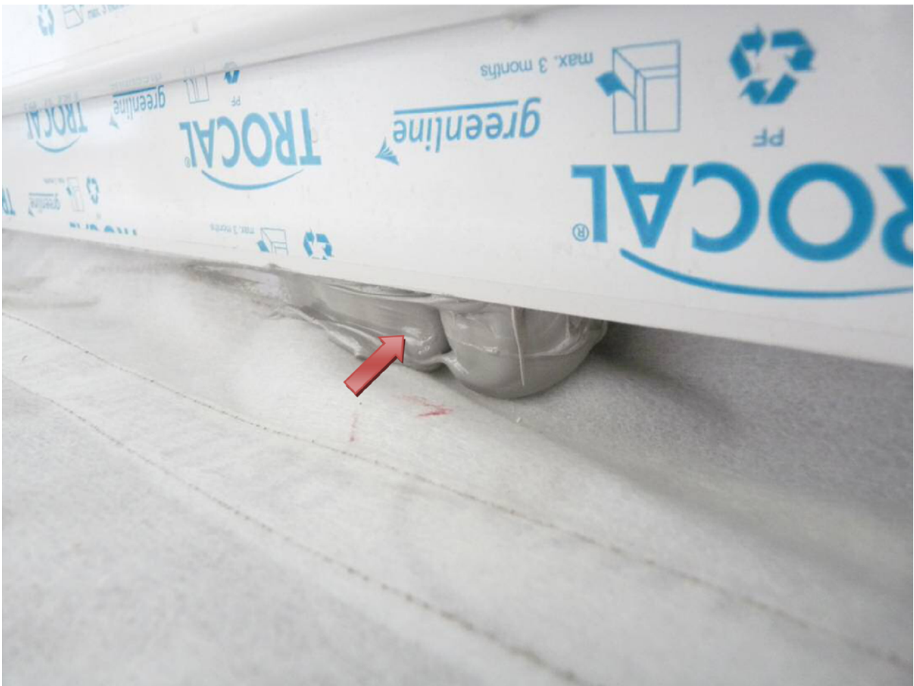
Abdichtung Innenseite
